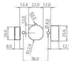
Pannello di montaggio Mounting template
